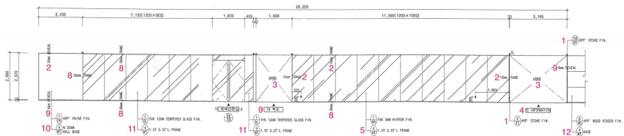
지하 2층 피트니스 센터 입면 F' / B2 floor fitness center elevation F'
