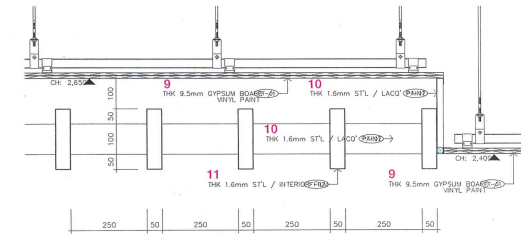
부페 천정 단면 상세 / buffet restaurant ceiling section
