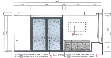
J 타입 내실 입면 V / J type room elevation V
