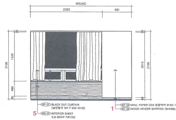
D 타입 내실 일면 O / D type room elevation O
