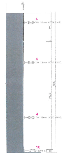
기둥 단면 상세 h / column section h
