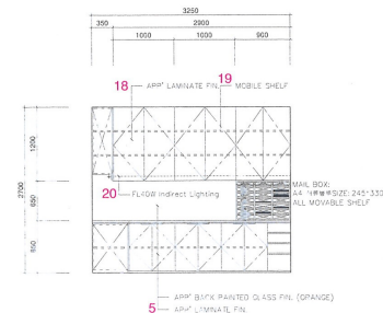
탕비실 입면 G / canteen elevation G
