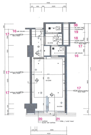
호텔 A 타입 실 천장 / A type room ceiling plan
