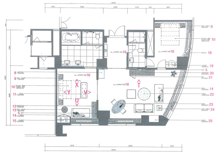
호텔 J 타입 실 평면 / hotel J type room floor plan
