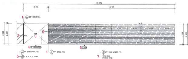
지하 2층 피트니스 센터 입면 F / B2 floor fitness center elevation F
