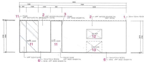
리셉션 입면 C / reception elevation C
