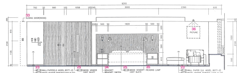
A 타입 객실 일면 J / A type room elevation J
