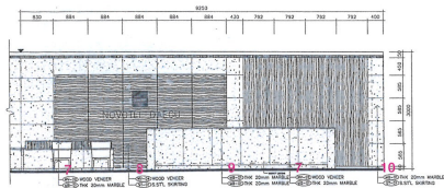
로비 입면 B / lobby elevation B
