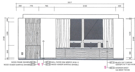
D 타입 내실 일면 N / D type room elevation N
