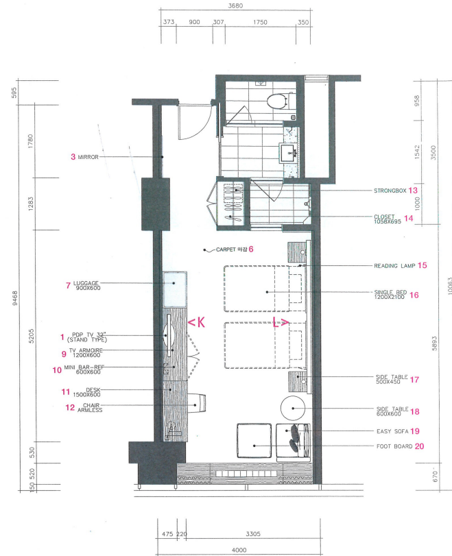
호텔 F 타입 실 평면 / hotel F type room floor plan
