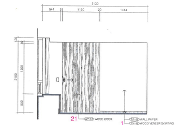
D 타입 내실 일면 S / D type room elevation S
