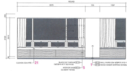
D 타입 내실 일면 R / D type room elevation R
