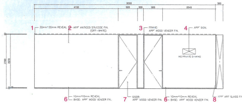
리셉션 입면 A / reception elevation A
