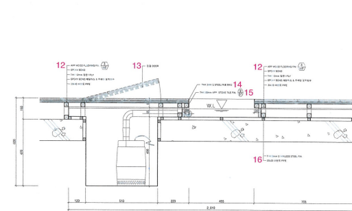
연못 단면 T / pond section T
