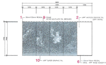
리셉션 입면 B / reception elevation B
