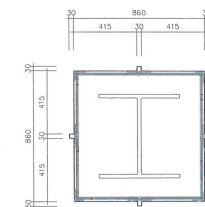
기둥 단면 상세 f / column section f
