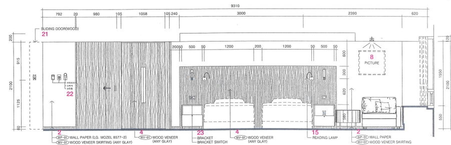
F 타입 내실 입면 L / F type room elevation L
