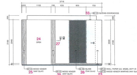
A 타입 객실 일면 G / A type room elevation G
