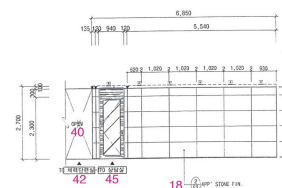
지하 2층 홀 입면 D / B2 floor hall elevation D
