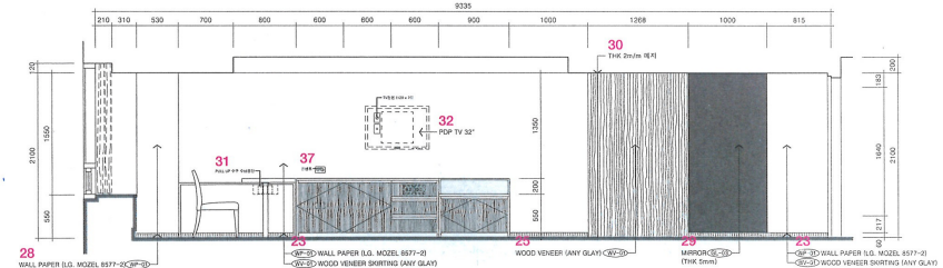
A 타입 객실 일면 I / A type room elevation I
