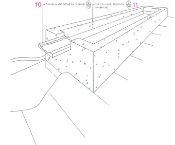
연못 투시도 / pond perspective
