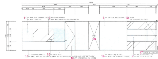
업무공간 입면 K / work area elevation K
