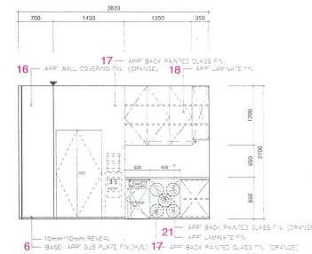
탕비실 입면 F / canteen elevation F
