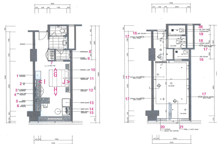
호텔 A 타입 실 평면 / A type room floor plan
