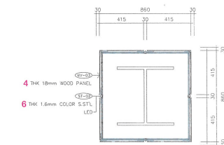
기둥 단면 상세 g / column section g
