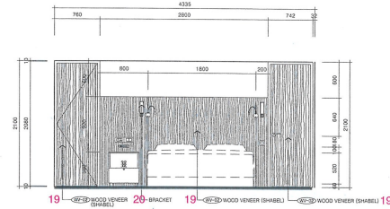
D 타입 내실 일면 P / D type room elevation P
