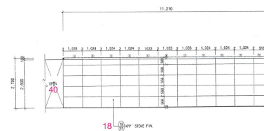
지하 2층 홀 입면 A / B2 floor hall elevation A
