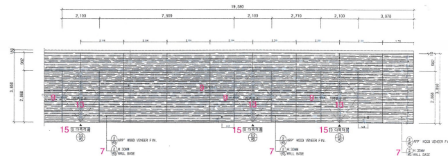
지하 1층 홀 입면 G' / B1 floor hall elevation G'
