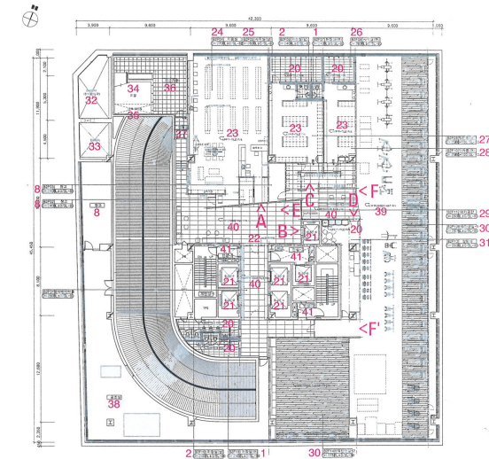
지하 2층 평면도 / B2 floor plan
