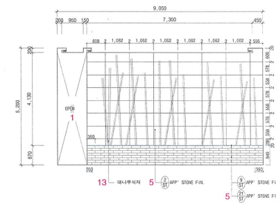
1층 라운지 입면 R / 1st floor lounge elevation R
