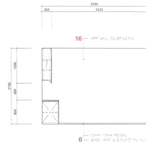
탕비실 입면 H / canteen elevation H
