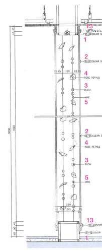
실내장식 단면 상세 d / decoration section d
