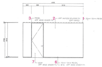
리셉션 입면 D / reception elevation D
