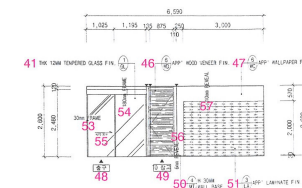
지하 2층 홀 입면 E / B2 floor hall elevation E
