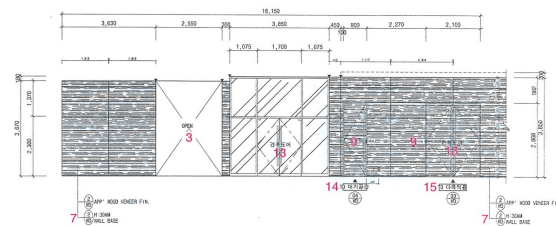
지하 1층 홀 입면 G / B1 floor hall elevation G
