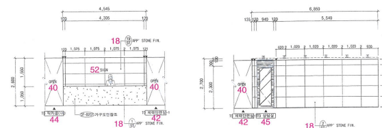
지하 2층 홀 입면 C / B2 floor hall elevation C
