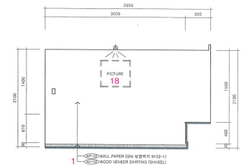
D 타입 내실 일면 Q / D type room elevation Q
