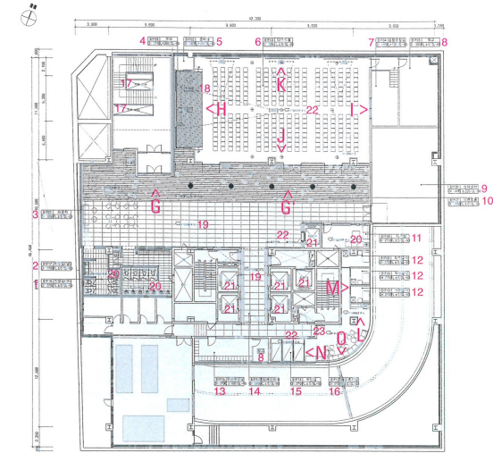
지하 1층 평면도 / B1 floor plan
