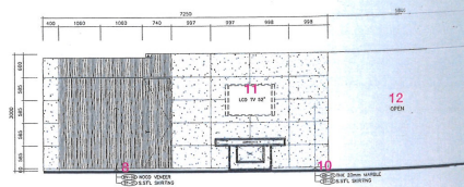
로비 입면 C / lobby elevation C
