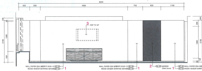
D 타입 내실 일면 M / D type room elevation M
