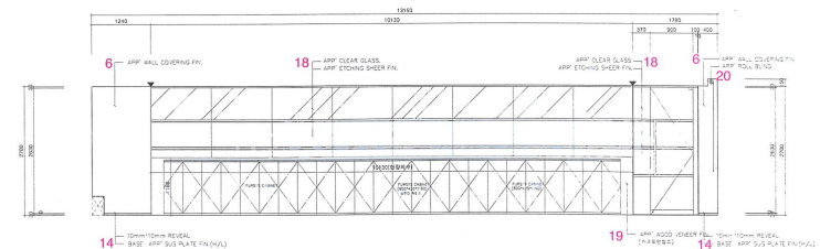
업무공간 입면 L / work area elevation L
