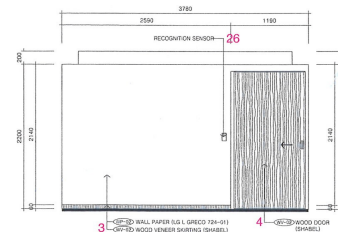
J 타입 내실 입면 X / J type room elevation X
