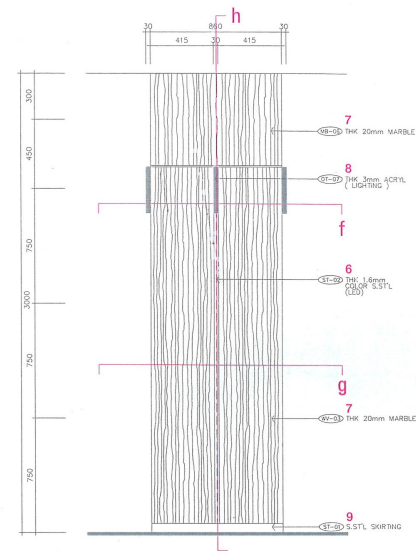
부페 기둥 e / buffet restaurant column e
