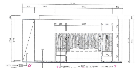
J 타입 내실 입면 Y / J type room elevation Y
