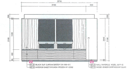
A 타입 객실 일면 H / A type room elevation H
