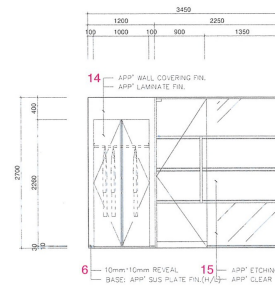
탕비실 입면 E / canteen elevation E
