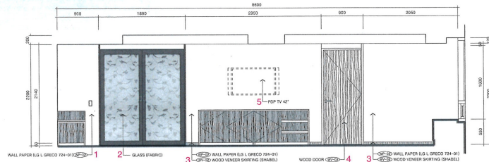
J 타입 내실 입면 T / J type room elevation T
