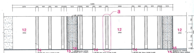
로비 입면 A / lobby elevation A
